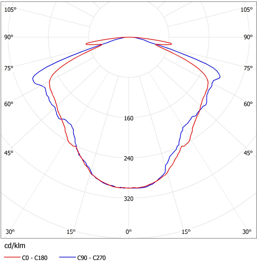
Кривая распределения сил света для светильника COSMO DELTA LED
