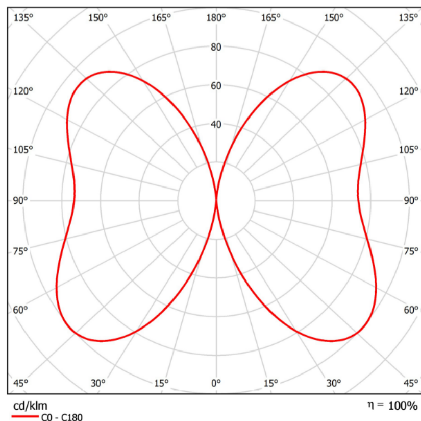
Кривая сил света КАРИН ДЕКОР 2400 LED
