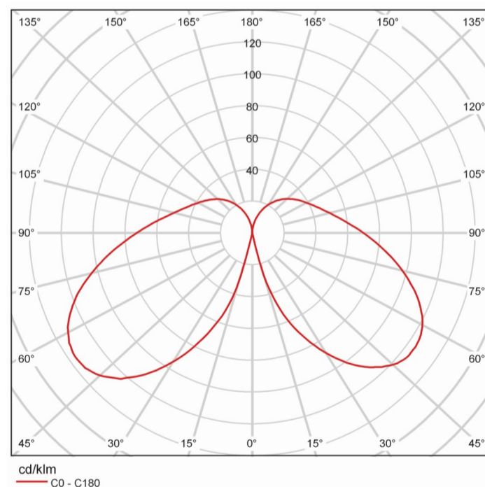
Кривая сил света КАРИН 600 LED
