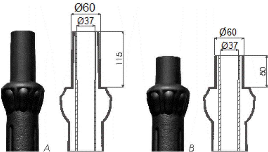
Сечение окончаний опор
