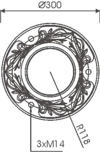
Основание опоры
